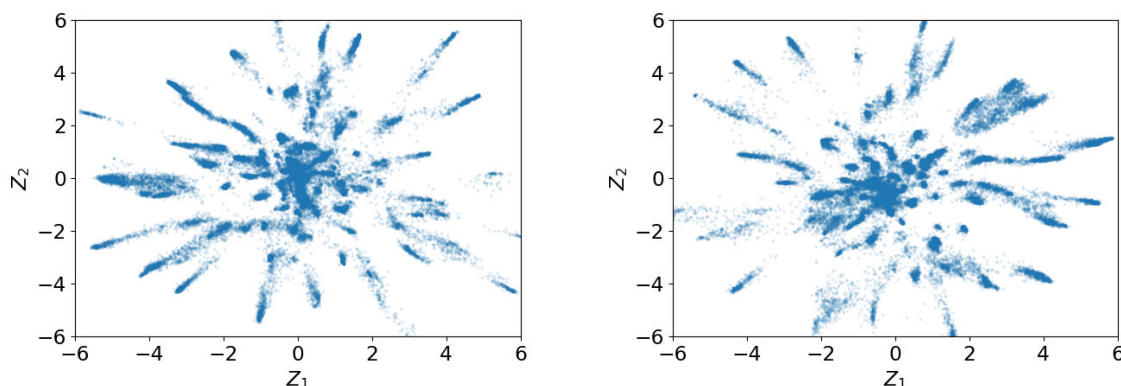
Obrázek 8.2: Latentní prostor pro query sekvenci PIP_BREBN/26-275 s ponechánými mezerami ( vlevo ) a bez mezer ponechaných mezer mimo pozice query sekvence ( vpravo ).
