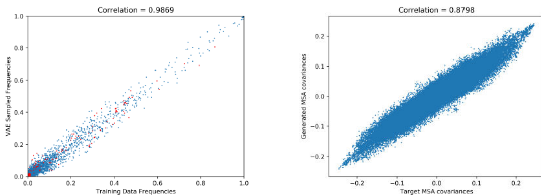
Obrázek 8.11: Statistiky prvního a druhého řádu pro konečný model s jednou skrytou vrstvou s 450 neurony vybraného pro experiment. Vlevo: statistika prvního řádu s vysokou korelací značí schopnost VAEs reflektovat frekvence aminokyselin na daných pozicích. Vpravo: korelace kovariance statistik druhého řádu.
