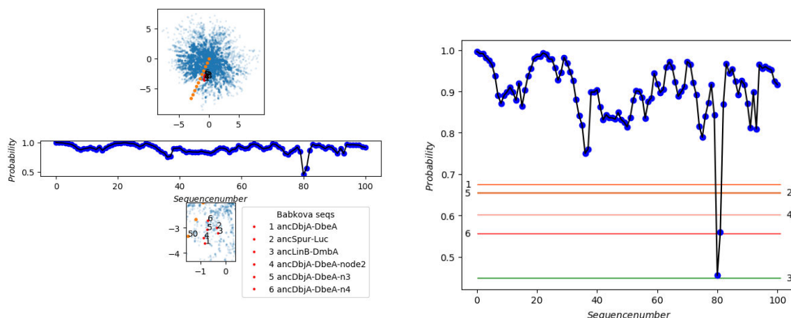
Obrázek 8.7: Statistický profil pozorovaných sekvencí strategie přímé evoluce. Vlevo: latentní prostor experimentu včetně pozic vygenerovaných sekvencí. Sekvence Babkové jsou zarovnány a zobrazeny v latentním prostoru, kde jsou umístěny blízko středu evoluční trajektorie. Vpravo: detail profilu sekvencí společně s pravděpodobnostními hodnotami pro sekvence Babkové.
