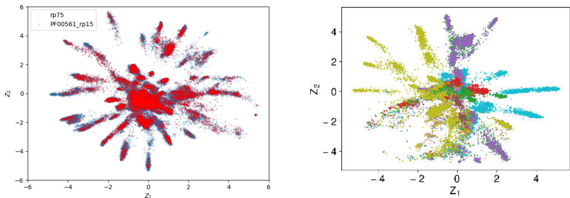
Obrázek 8.4: Latentní prostor dobře reflektuje podvzorkovací proces v RPXX Pfam podrodinách ( vlevo ). Fylogenetický strom pro PF00561 namapován do latentního prostoru pro jednotlivé evoluční větve ve zkoumaný evoluční okamžik ( vpravo ).
