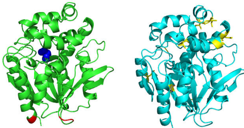
Obrázek 8.8: Příklady přímých předků vygenerovaných na základě latentního prostoru pro DhaA . Vlevo: Varianta AncDhaA16 s identitou 69,23 % pouze zvýrazněné pozice inserce/delece, červeně - delece (dvě ve smyčce, pozice 29 a 30, a jedna ve šroubovici, pozice 291), modře - inserce S (jedna ve smyčce, pozice 133). Vpravo: Varianta AncDhaA7 s 93,89% identitou WT. Všech 10 navržených záměn je zvýrazněno.
