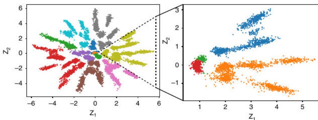
Obrázek 5.3: Latentní prostor zachycuje evoluční vztahy v proteinových rodinách. Barevně shodné body odpovídají sekvencím patřícím do stejné podvětvě fylogenetického stromu. Řez stromu je proveden v určité hloubce odpovídající zkoumanému času evoluce. Vpravo: variační autoenkodér je schopný zachytit evoluční vztahy i na detailnějším podprostoru fylogenetického stromu. Převzato z [14].
