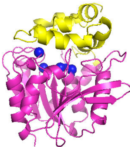
Obrázek 6.1: Zástupce rodiny haloalkan dehalogenáz protein 1bn6 [49]. Hlavní doména je zvýrazněna růžově, víčková žlutě. Modré kuličky značí katalytické residua proteinu.
