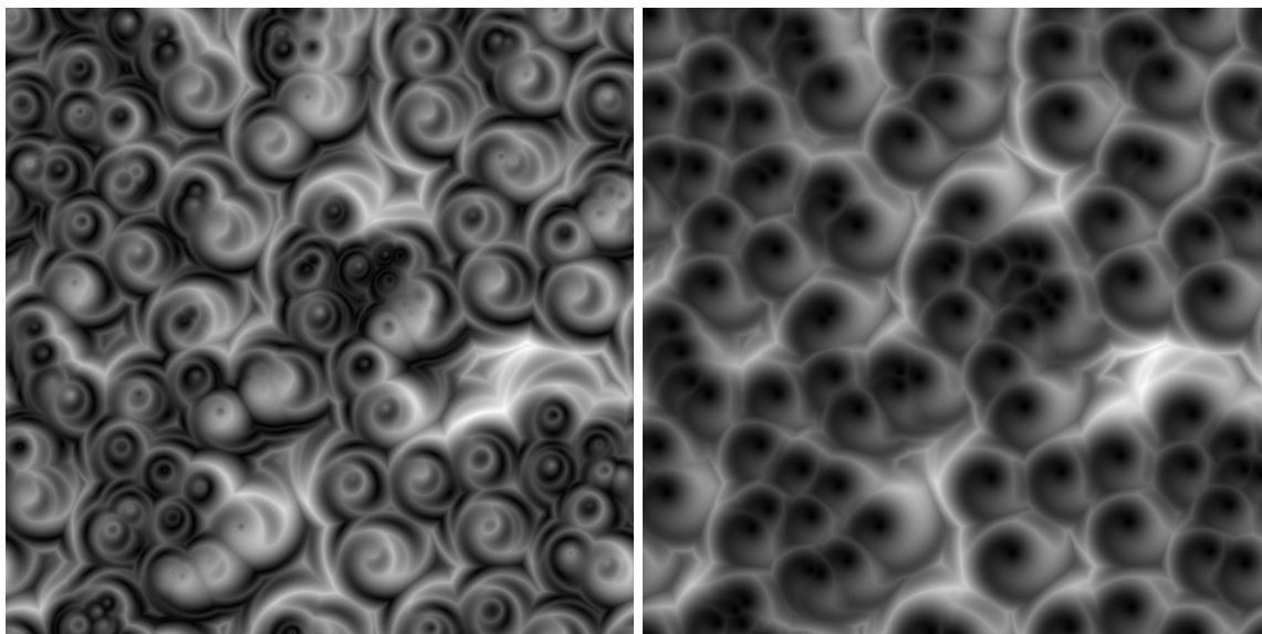
Obrázek 3.10: Lokální transformace
