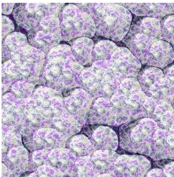
Obrázek 3.11: Sestavená textura
