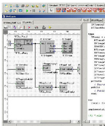
Obrázek 13: Grafický editor OpenWire ve vývojovém prostředí Delphi 7.
