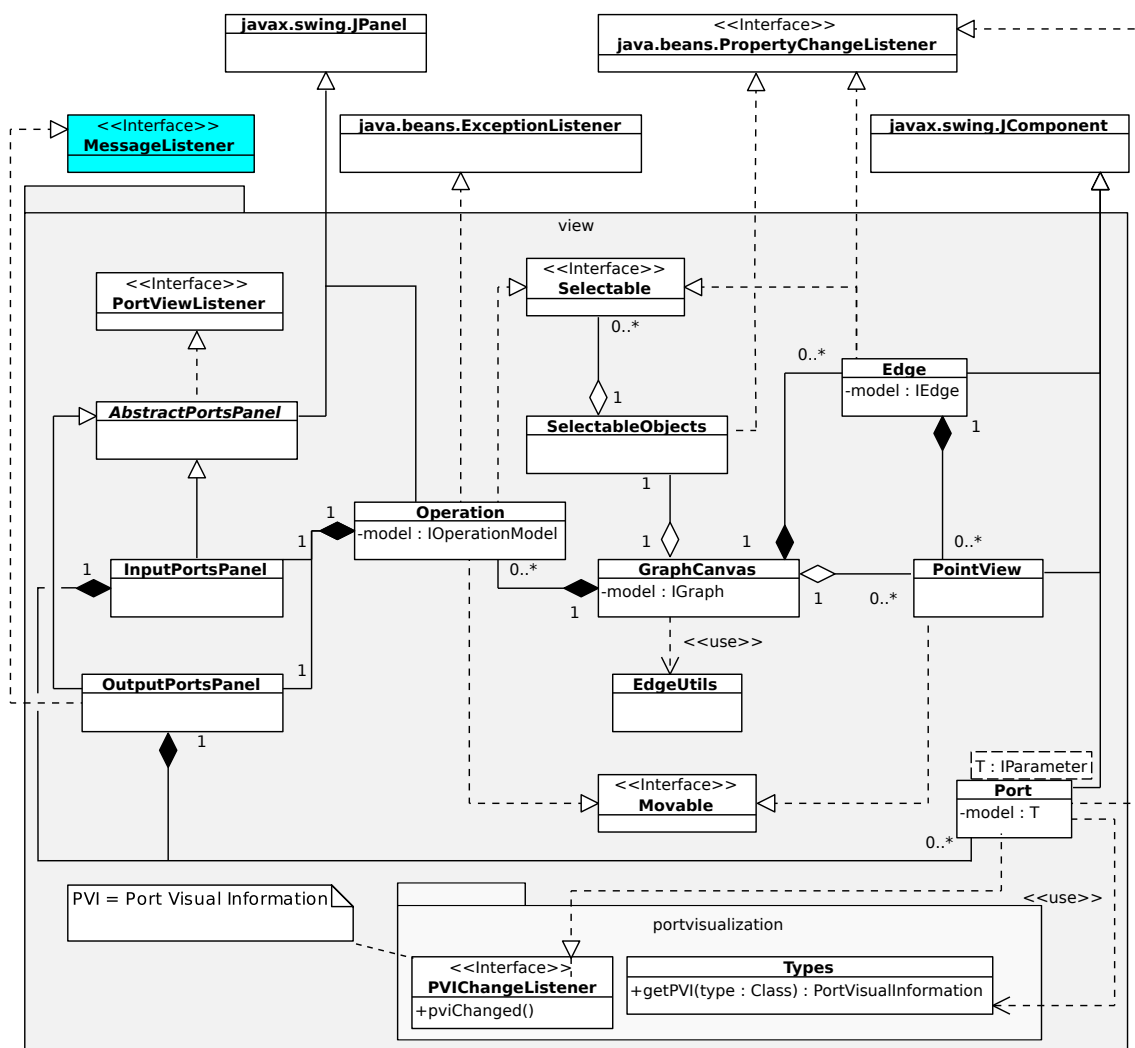
Obrázek 29: Pohled – struktura tříd.
