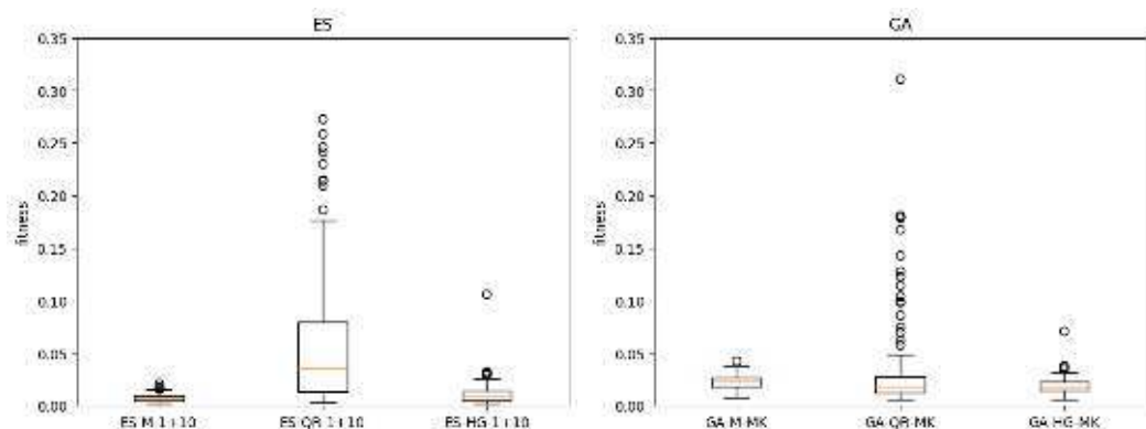
Obrázek 6.19: Experiment 4 varianta Cloning. Statistické zhodnocení experimentů. Zleva evoluční algoritmus ES, GA.
