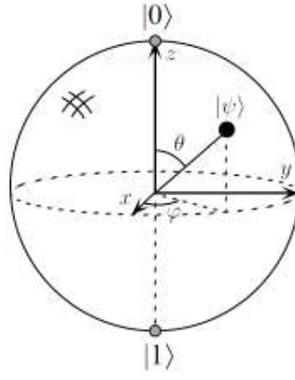
Obrázek 2.2: Blochova sféra [37].
