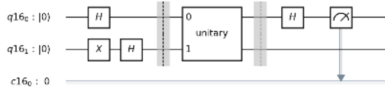
Obrázek 2.9: Deutschův algoritmus [37].
