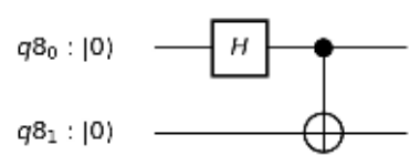
Obrázek 2.8: Obvod kvantového provázání
