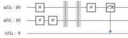
Obrázek 2.10: Deutschův algoritmus s hradlem U_f pro f(x) = 0
