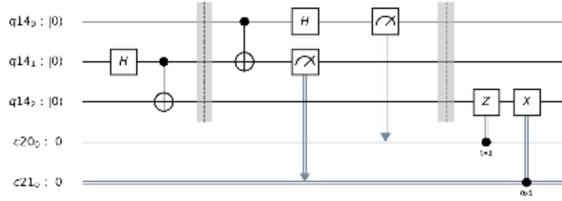
Obrázek 2.15: Obvod Teleportace [37].
