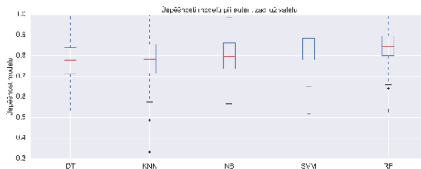
Obrázek 5.7: Rozdělení úspěšností modelů při autentizaci jednotlivých uživatelů.
