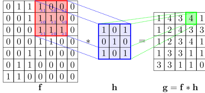
Obrázek 5.5: Příklad diskrétní konvoluce 5 .
