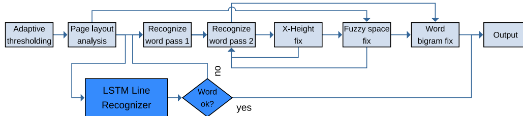
Obrázek 6.5: Architektura Tesseract-OCR 3 .
