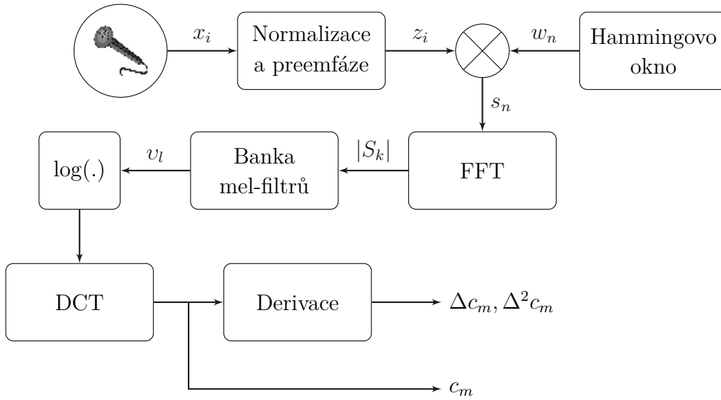
Obrázek 4.4: Schéma výpočtu mel-frekvenčních keprstrálních koeficientů.
