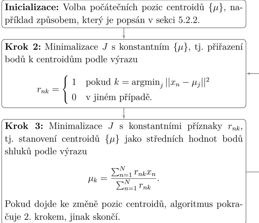
Obrázek 5.2: Schéma průběhu algoritmu K-means.
