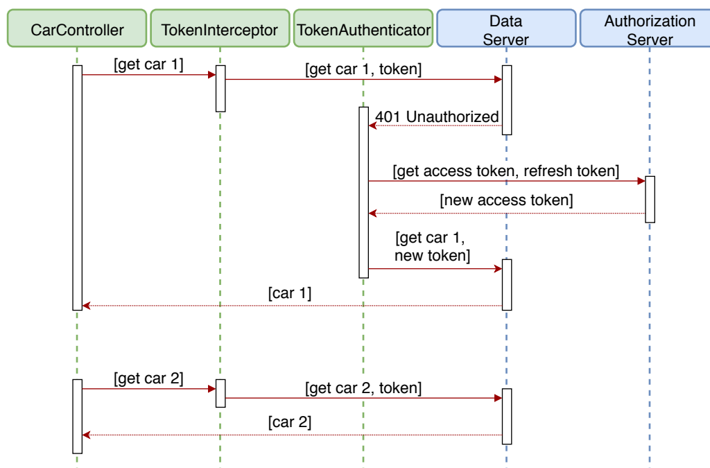
Obrázek 5.2: Sekvenční diagram automatické správy tokenů v požadavcích za použití tříd TokenInterceptor a TokenAuthenticator . V prvním požadavku vypršela autorizačnímu tokenu platnost a je zažádáno o nový. Ve druhém požadavku je již autorizační token platný a data jsou získána ihned.
