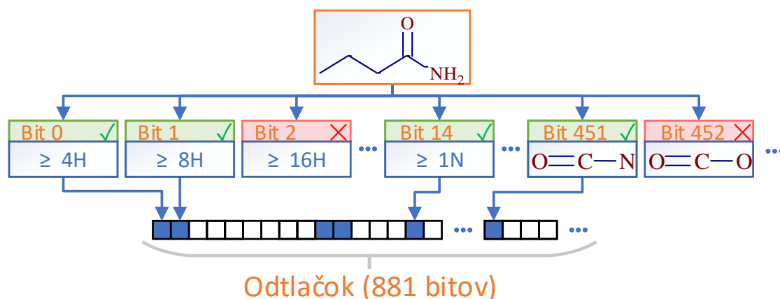
Obr. 3.5: Princíp vytvárania CACTVS odtlačku na niekoľkých vybraných bitoch. Znázorňované bity 451 a 452 sú pomocou jazyka SMARTS popísané ako C(-N)(=O) a C(-O)(=O) .
