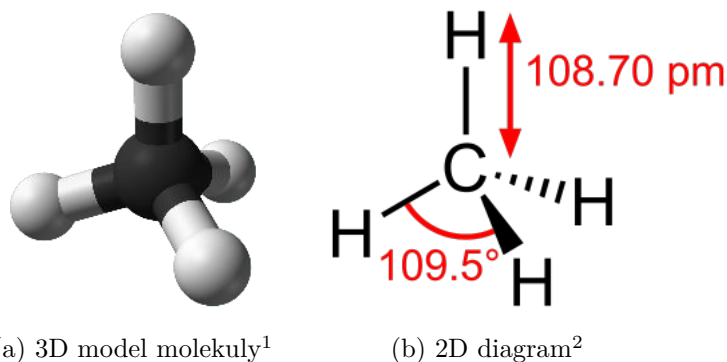
Obr. 2.8: Priestorová reprezentácia molekuly metánu
