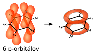
Obr. 2.9: Orbitály v benzéne 3
