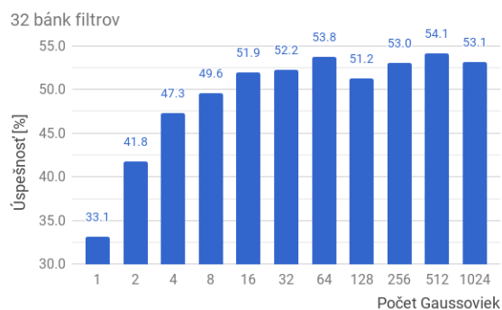
(d) 32 bank filterov
