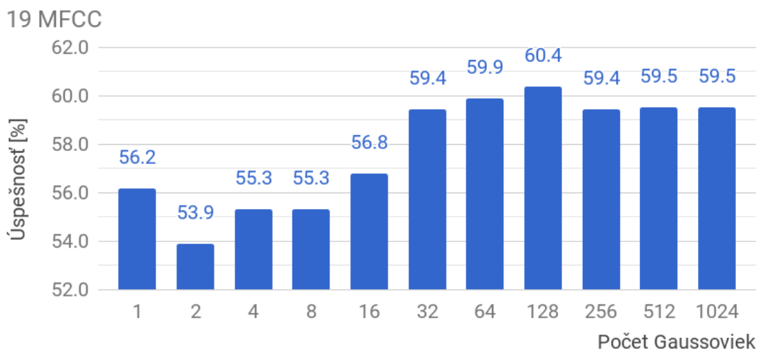
(a) Najlepší GMM systém s 19 MFCC koeficientami.
