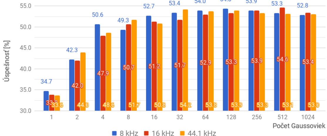
(c) Systémy so 44 bankami filtrov.
