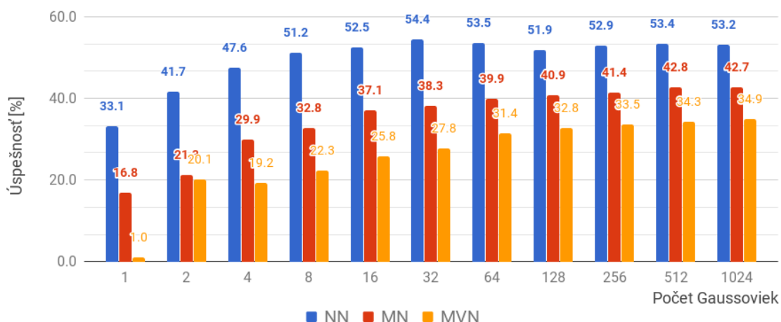
(a) Systémy s 20 bankami filtrov.
