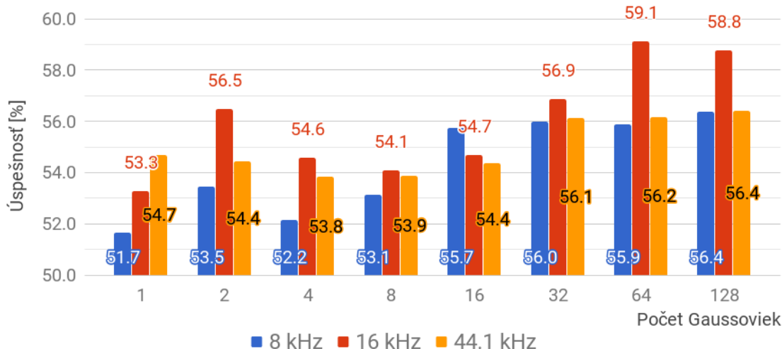
(b) Systémy s 20 MFCC koeficientami.
