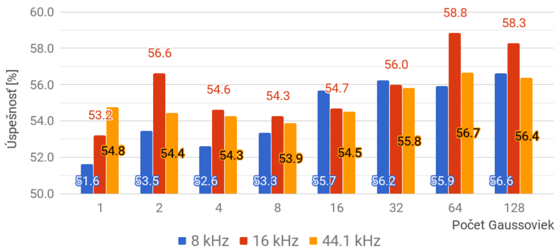
(a) Systémy s 19 MFCC koeficientami.
