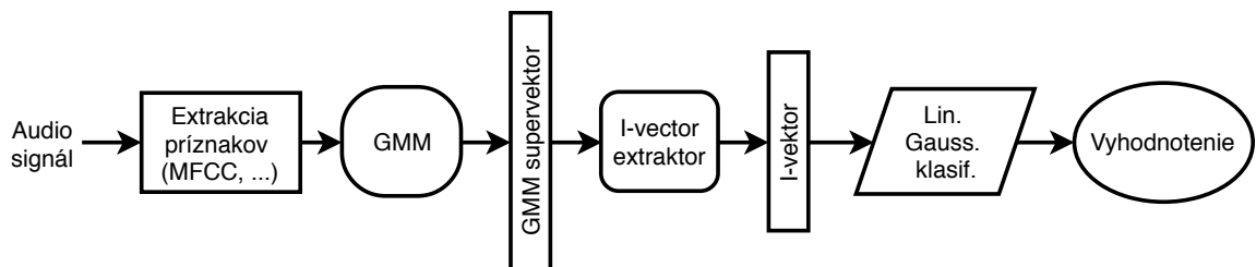
Obr. 3.3: Bloková schéma i-vektor systému.
