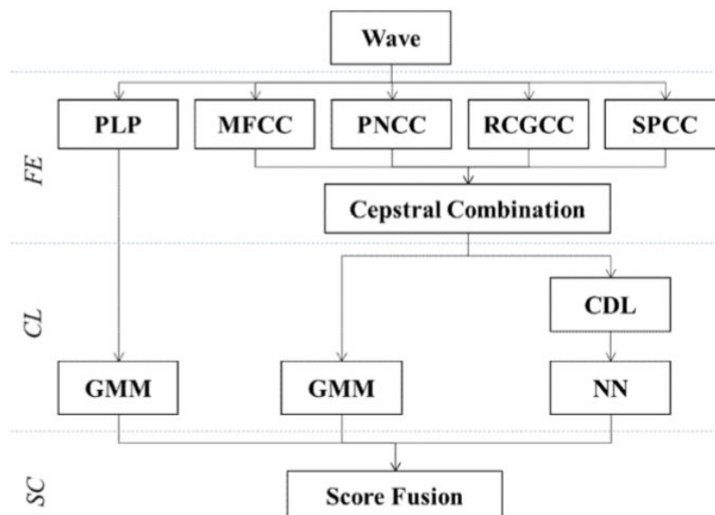
Obr. 2.5: Architektúra úspešného kórejského systému pre klasifikáciu akustického prostredia ( FE=Feature Extraction , CL=Classification , SC=Score Fusion ). Obrázok prevzatý z [20].
