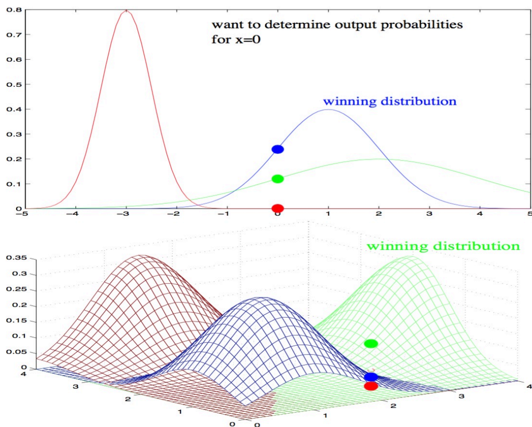
Obr. 3.5: Ilustrácia modelovania jednotlivých tried pomocou jednorozmerných (hore) a dvoj-rozmerných (dole) Gaussovských rozložení [23].
