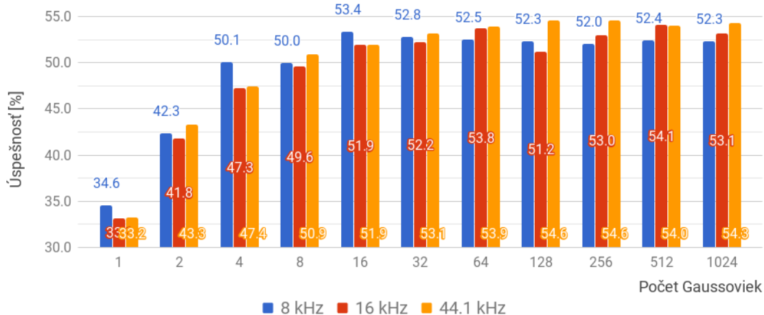
(b) Systémy s 32 bankami filtrov.
