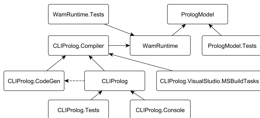
Obrázek 6.1: Závislost jednotlivých projektů v rámci implementace
