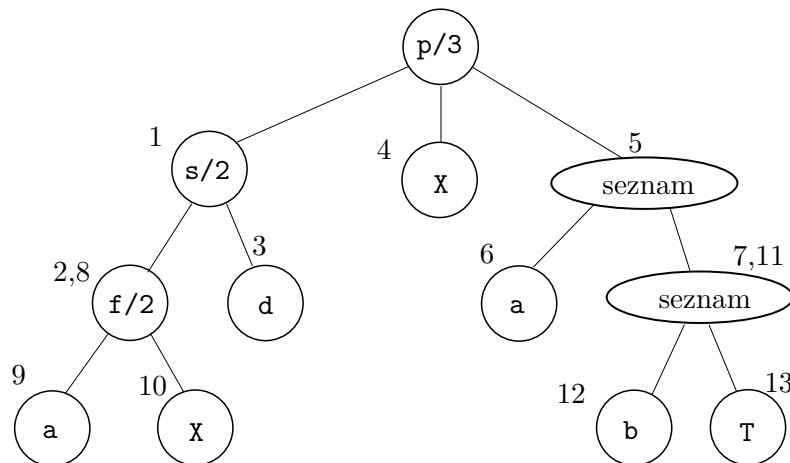
Obrázek 6.5: Pořadí průchodu uzly hlavičky p(s(f(a,X),d), X, [a,b|T]) při překladu
