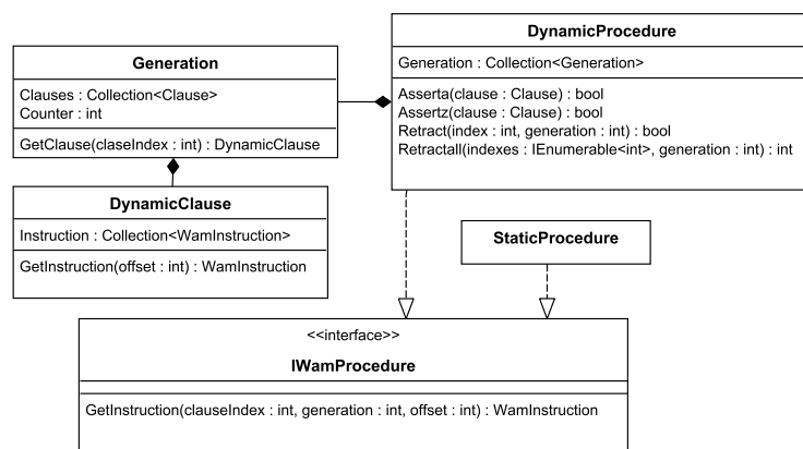
Obrázek 5.1: UML diagram vnitřní reprezentace procedur
