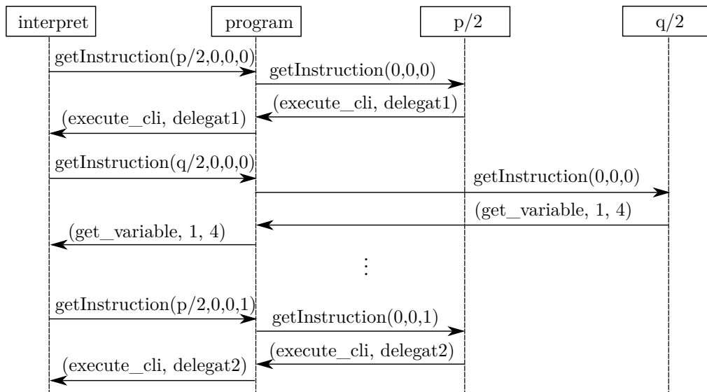
Obrázek 5.3: Diagram volání při vyhodnocování vestavěného predikátu
