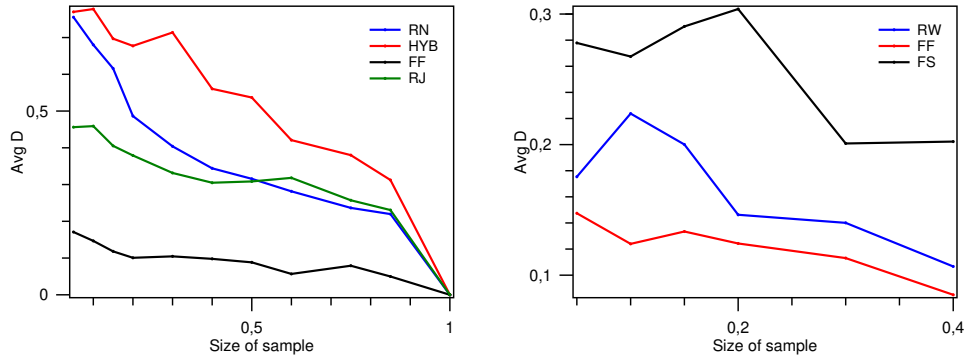
(a) RN, HYB, FF a RJ metoda - elektrická síť (b) RW, FF a FS metoda - DBLP síť
