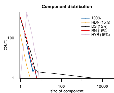
(a) distribuce velikost komponent
