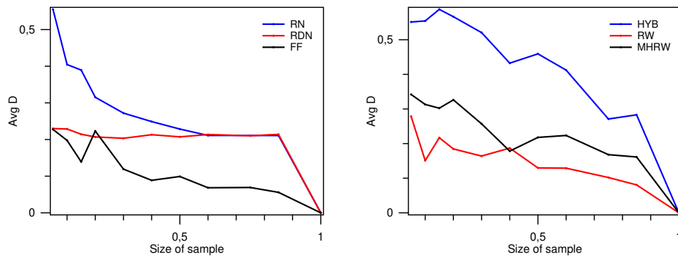
(a) porovnání metod založených na výběru vrcholů (RN, RDN) s FF metodou (b) porovnání metod založených na procházení grafu (RW, MHRW) s HYB metodou.
