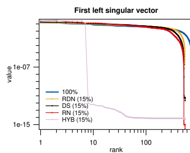
(e) První levý singulární vektor
