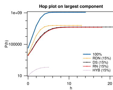
(c) Hop-plot na největší komponentě
