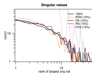
(f) Singulární hodnoty
