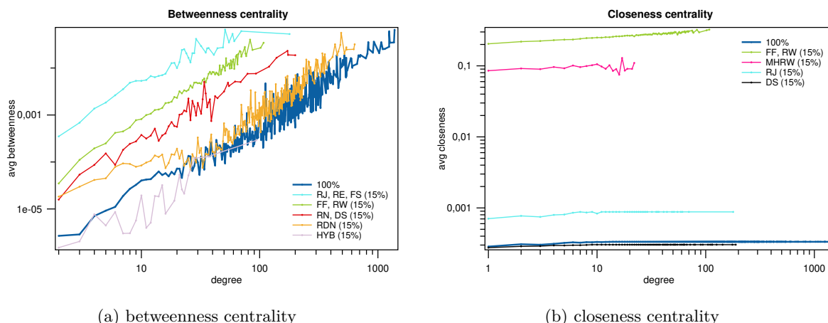
Obrázek 13: Distribuce centralit - Enron síť .
