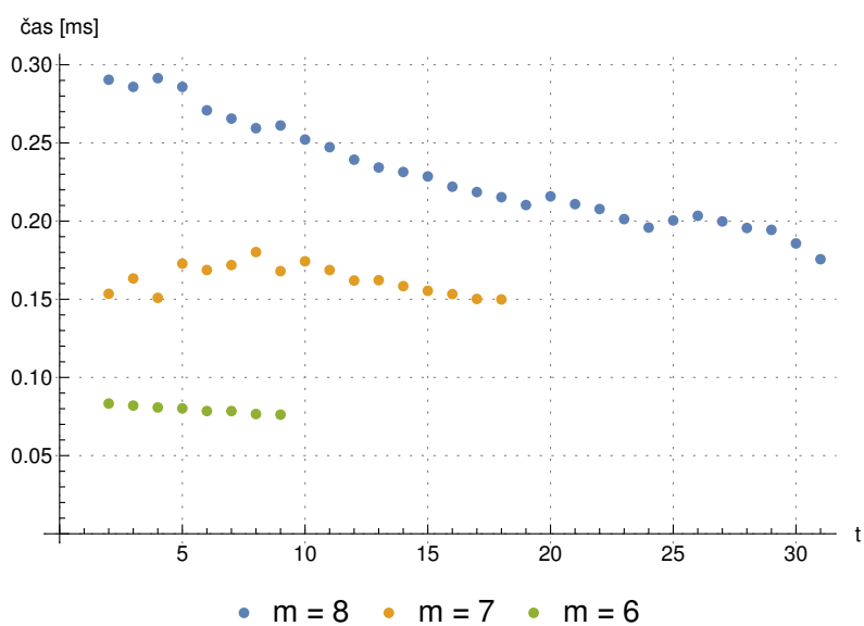
Obrázek 7.2: Závislost doby šifrování zprávy na parametru t (při různých volbách m )
