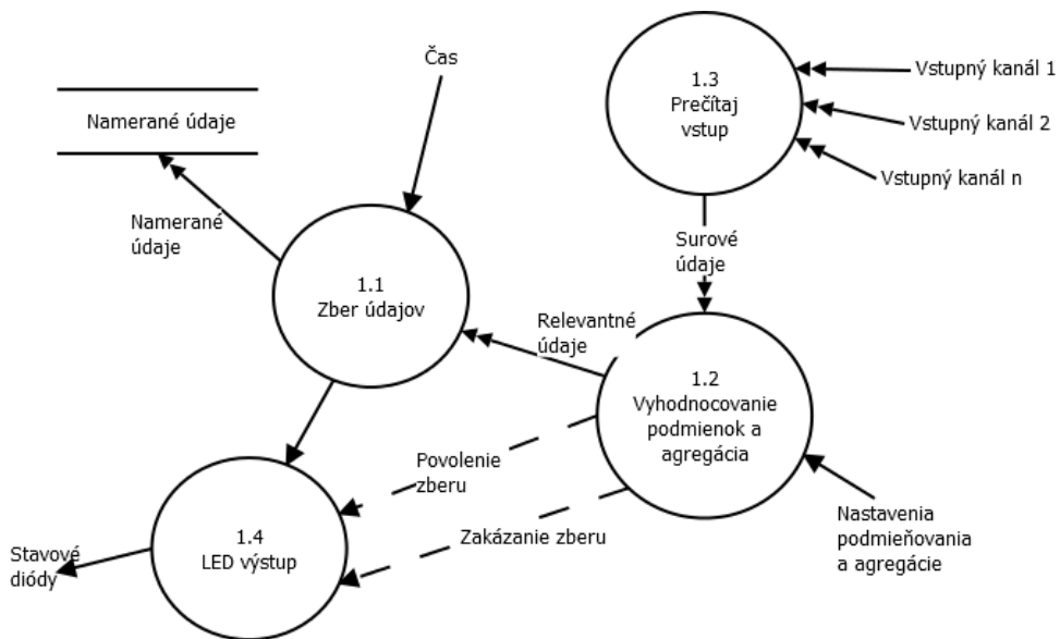
Obr. 15.: Vykonaj DAQ - transformácia.
