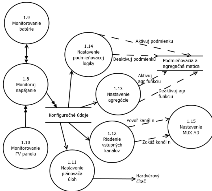
Obr. 17.: Vykonaj systémové nastavenie a kontrolu – transformácia.
