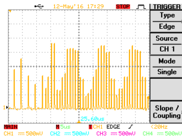
Obr. 19.: Priebeh hodinového signálu na karte SD.
