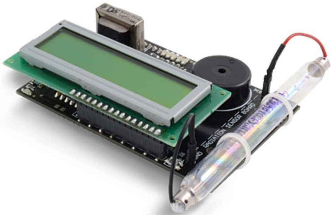
Obr. 26.: Radiačný senzor s trubicou J305 \beta
