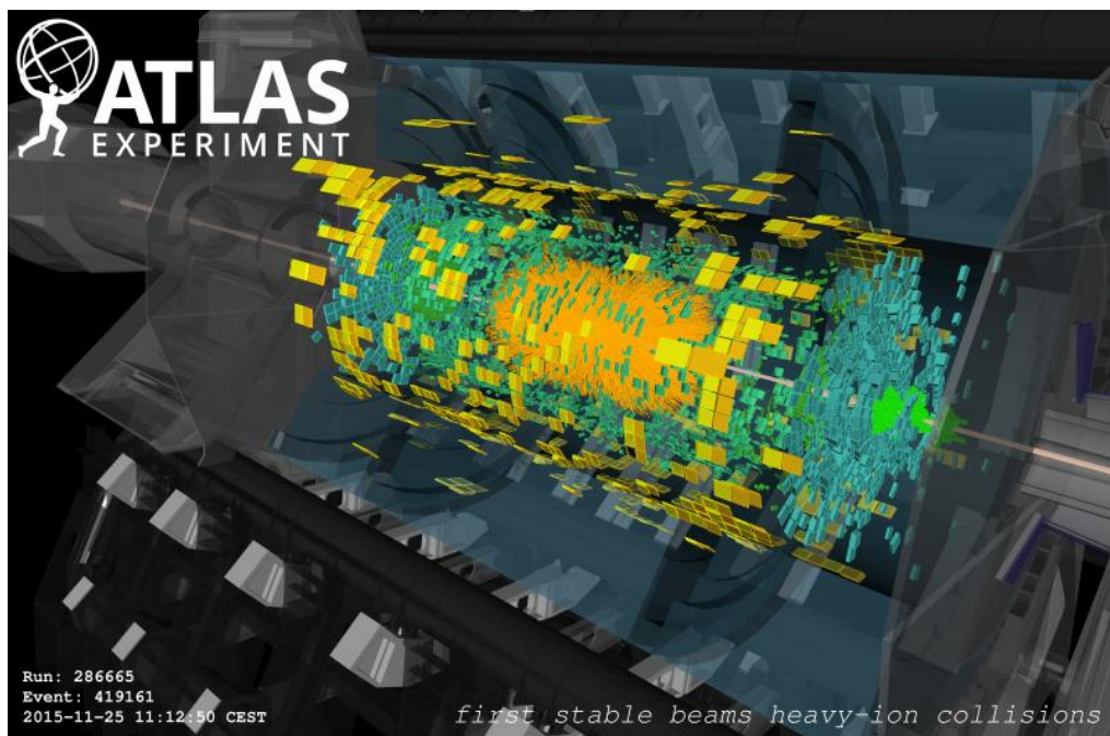
Obr. 4.: Vizualizácia udalosti v detektore ATLAS.
