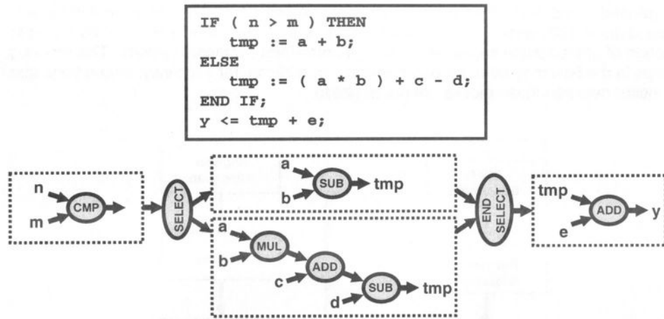
Obrázek 2.2: Příklad CDFG grafu vytvořeného z algoritmu. Převzato z [2].
