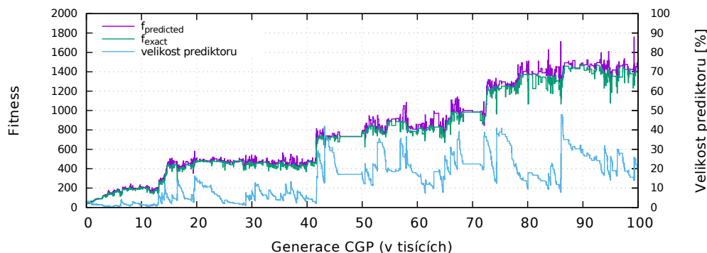
Obrázek 5.11. Průběh predikované a skutečné fitness a velikosti prediktoru pro jeden konkrétní běh s 15% šumem typu sůl a pepř
