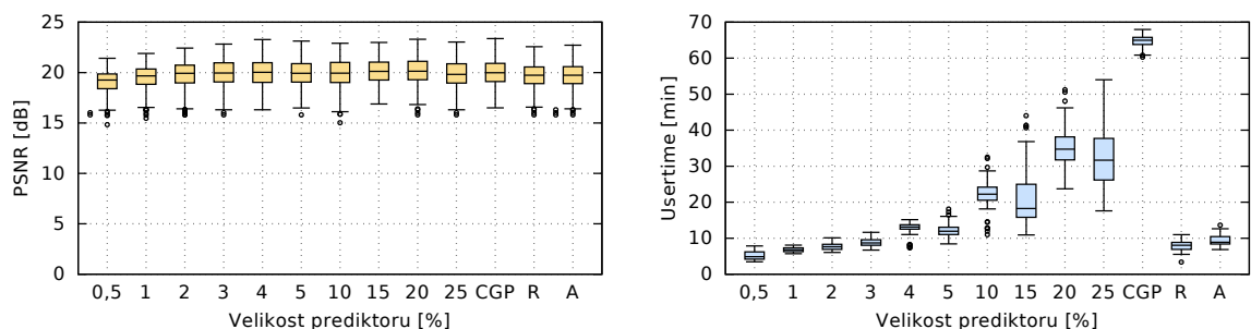
Obrázek B.23. 40% výstřelový (náhodný) šum
