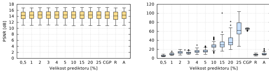
Obrázek B.29. 75% výstřelový (náhodný) šum
