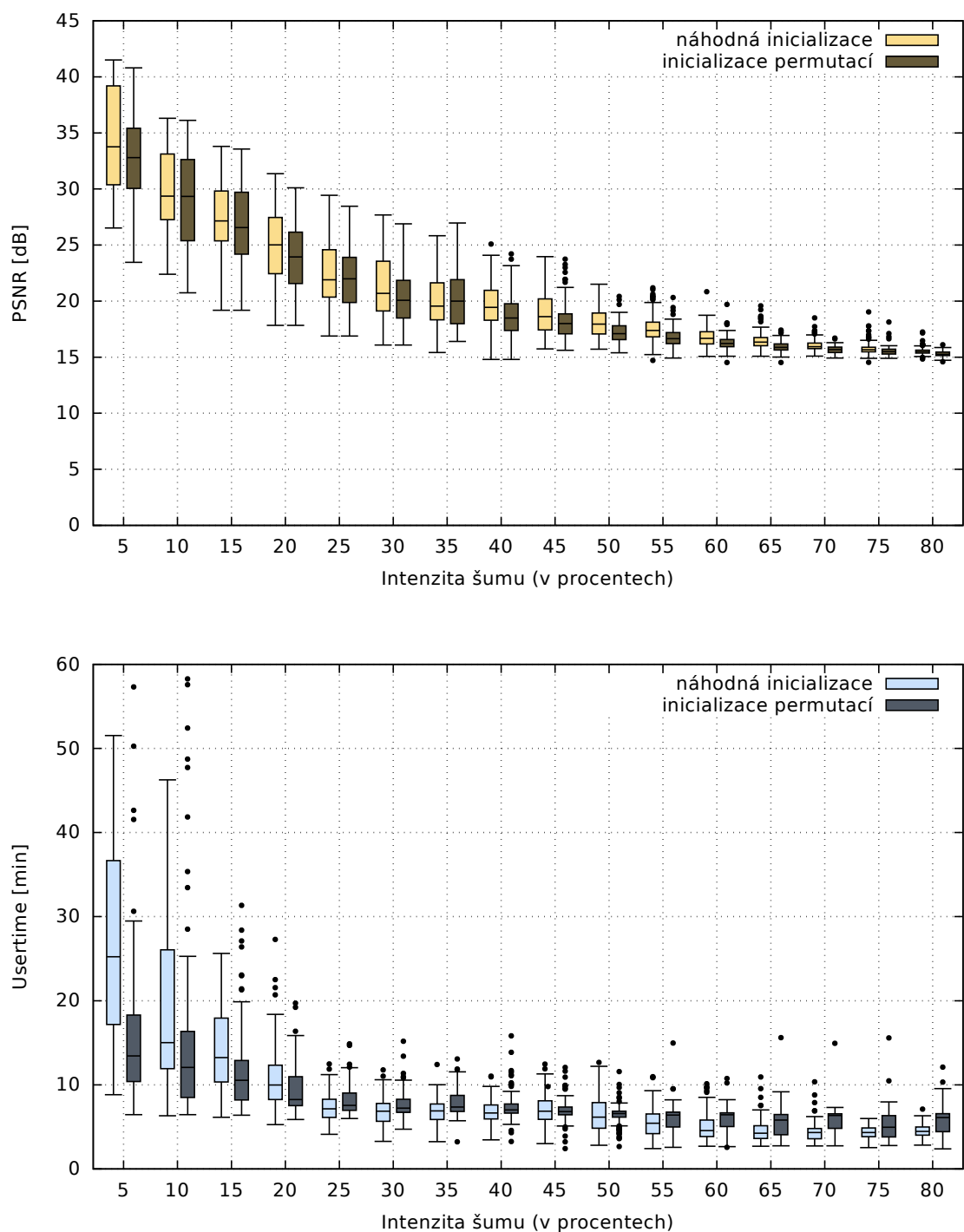
Obrázek 5.8. Vliv způsobu inicializace prediktorů fitness pro různé intenzity šumu typu sůl a pepř
