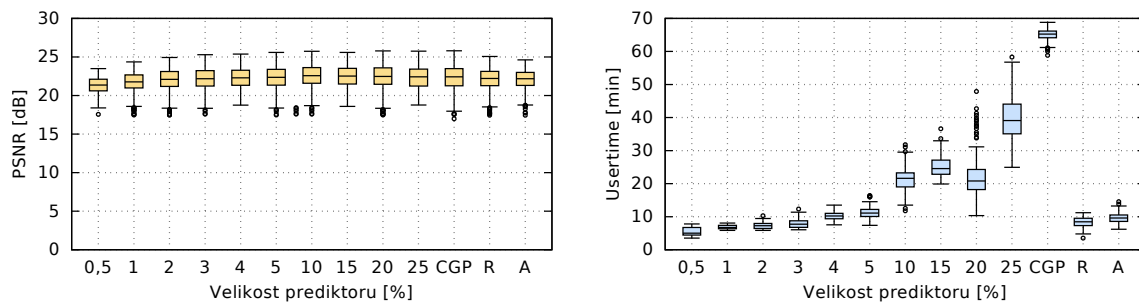
Obrázek B.21. 30% výstřelový (náhodný) šum
