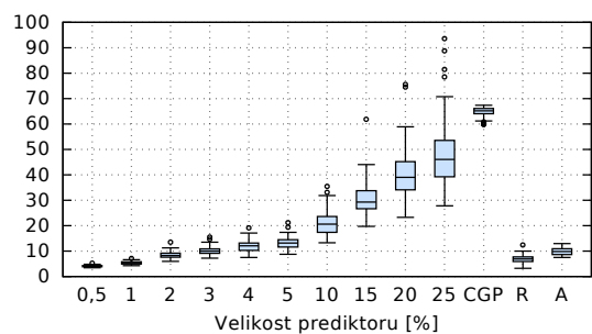
Obrázek B.7. 35% šum typu sůl a pepř
