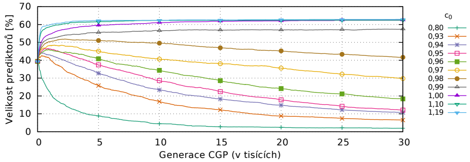
(b) Průběh velikosti prediktorů (průměr ze 100 běhů)
