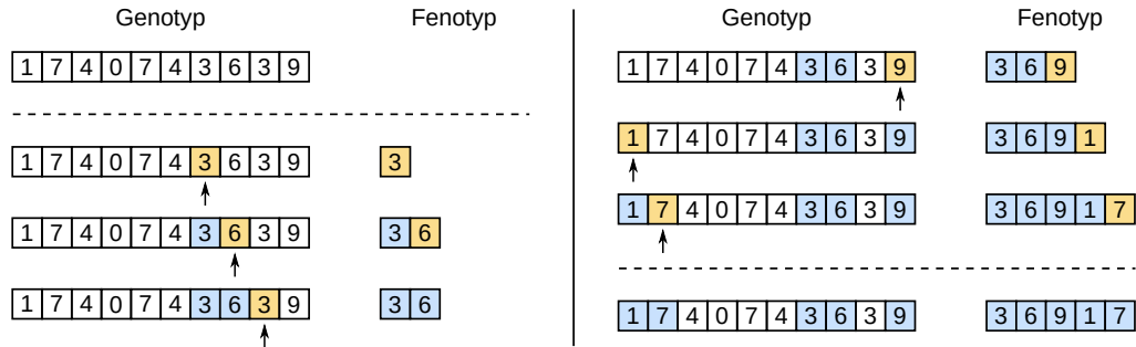
Obrázek 3.2. Postup konstrukce fenotypu prediktoru. Šipka označuje právě přečtený gen
