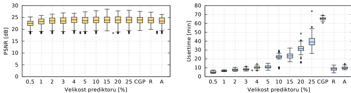
Obrázek B.20. 25% výstřelový (náhodný) šum
