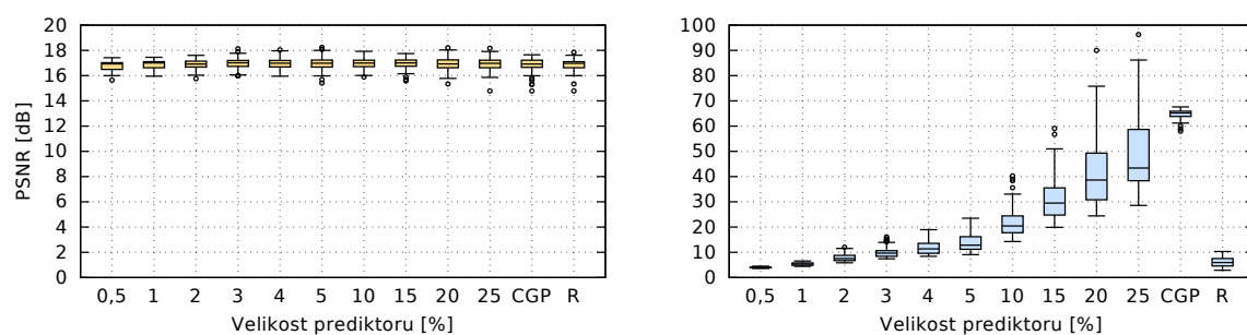
Obrázek B.31. Detektor hran
