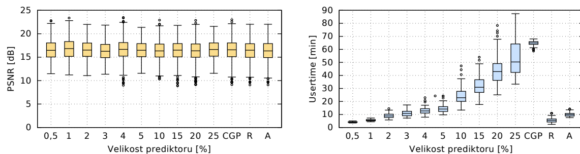
Obrázek B.11. 55% šum typu sůl a pepř
