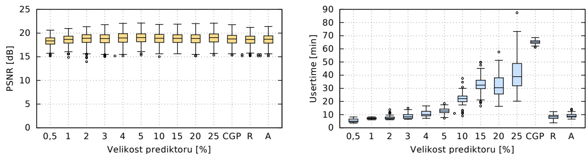
Obrázek B.24. 45% výstřelový (náhodný) šum
