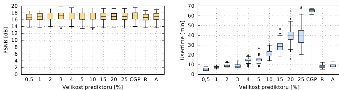
Obrázek B.26. 55% výstřelový (náhodný) šum
