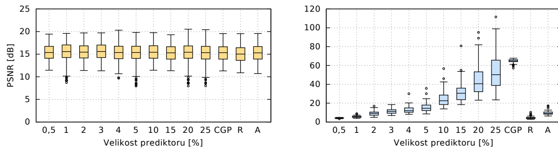
Obrázek B.13. 70% šum typu sůl a pepř
