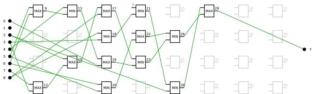
(d) Zapojení evolvovaného filtru
