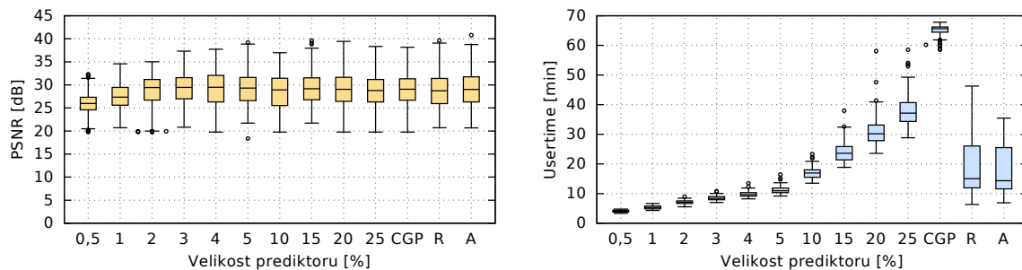
Obrázek B.2. 10% šum typu sůl a pepř
