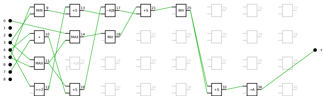
(d) Zapojení evolvovaného detektoru
