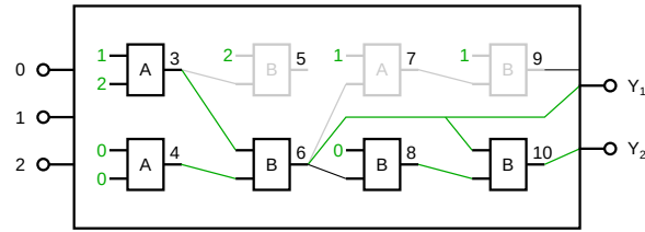
Obrázek 2.4. Program v kartézském genetickém programování. Uzly 5, 7 a 9 jsou neaktivní
