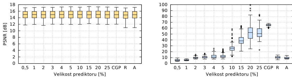
Obrázek B.28. 70% výstřelový (náhodný) šum
