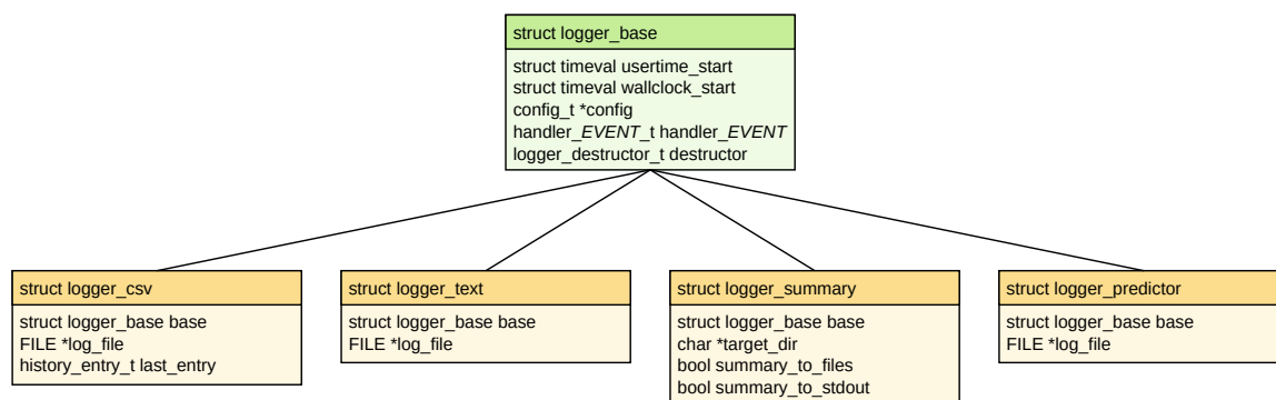
Obrázek 4.3. Datové typy modulů obsluhujících události a jejich hierarchie
