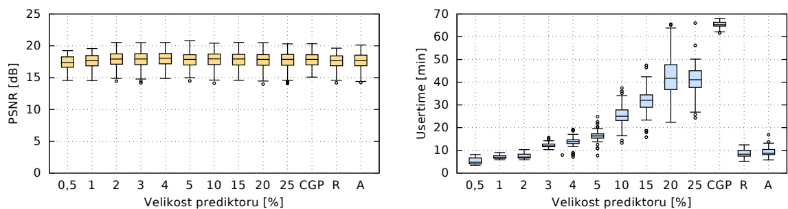
Obrázek B.25. 50% výstřelový (náhodný) šum
