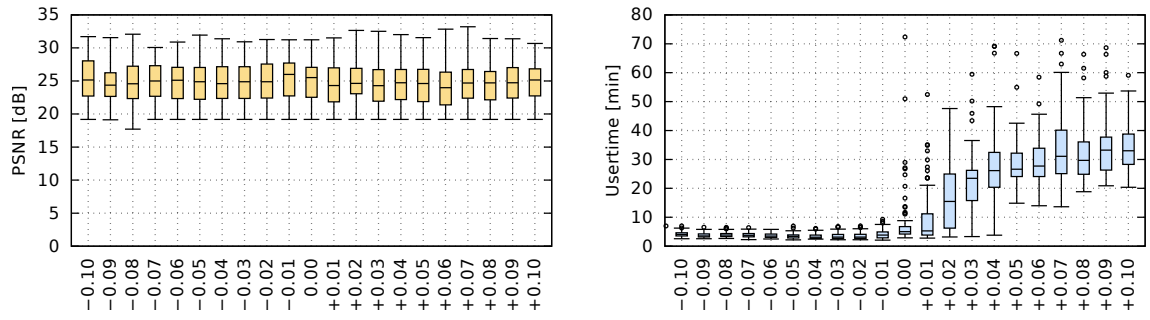
(a) Vliv parametru c_0 (pravidlo |v| \leq v_{zero} : UsedGenes \leftarrow UsedGenes + N \cdot c_0 )
