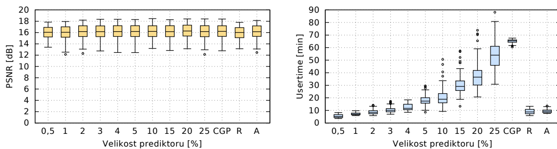
Obrázek B.27. 60% výstřelový (náhodný) šum
