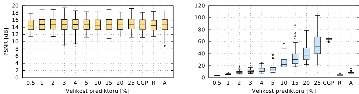
Obrázek B.15. 80% šum typu sůl a pepř
