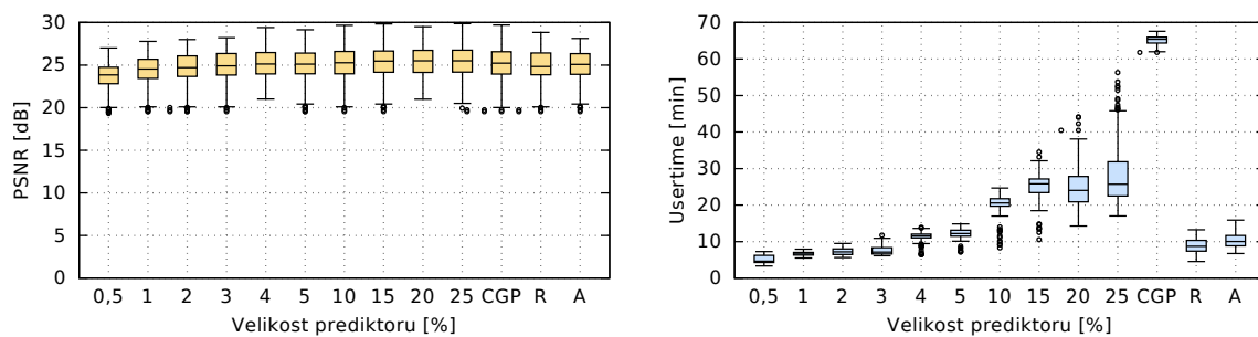
Obrázek B.19. 20% výstřelový (náhodný) šum
