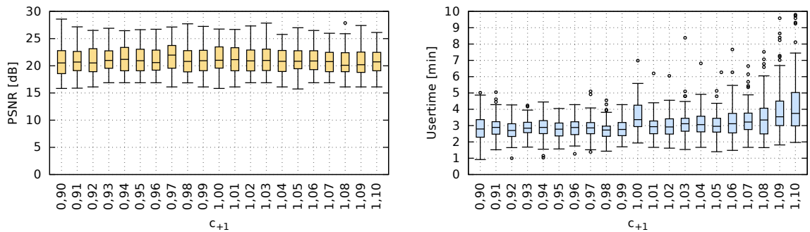
Obrázek 5.4. Vliv parametru c_{+1} (pravidlo 0 < v \leq v_{slow} : \text{UsedGenes} \leftarrow \text{UsedGenes} \cdot c_{+1} )
