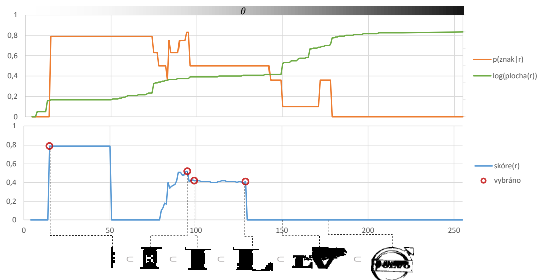
Obrázek 2.4. Sekvence p(\text{znak}|r) a \text{plocha}(r) , v logaritmickém měřítku podle prahu \theta . \text{skóre} = p \cdot (1 - a') v sekvenci inkluze extrémálních oblastí. Oblasti vybrané pro další fázi jsou označené kolečky.
