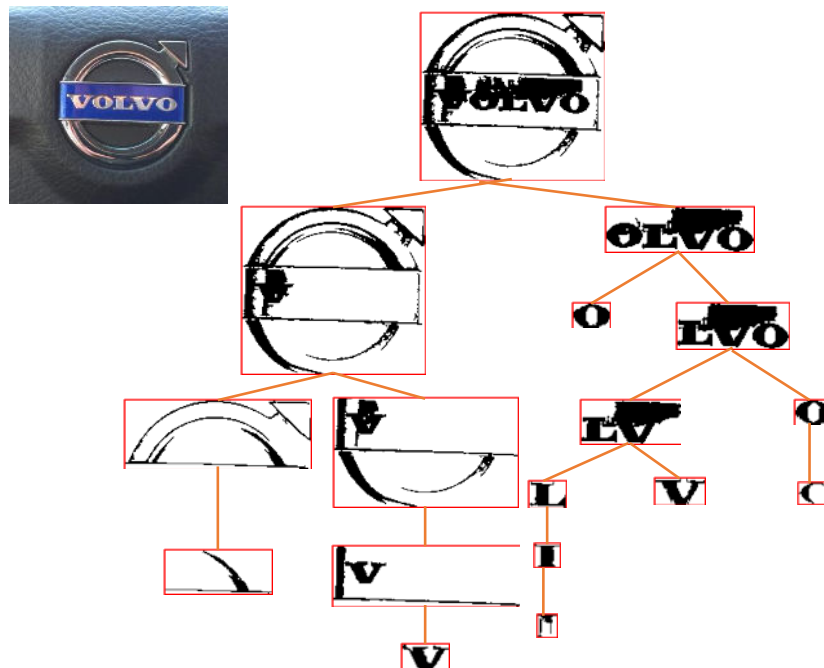
Obrázek 2.2. Některé extrémální oblasti v daném obrázku (reprezentovaným v negativu stupňů šedi); strom odpovídá skládání oblastí jako množin – nadřizený je nadmnožinou podřizného.
