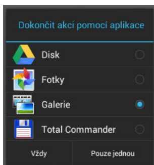
Obrázek 5.4. Klasický Intent pro výběr obrázku – souboru.
