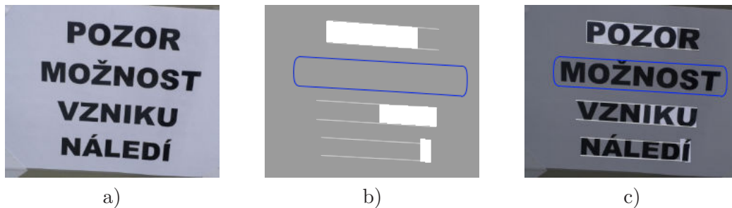
Obrázek 5.9. Ukázka (výřez) obsahu obou SurfaceView : a) spodní vrstva (původní obrázek), b) vrchní vrstva s animací 1 ). Zvýraznění pro POZOR ve fázi dorůstání , VZNIKU a NÁLEDÍ v 2. fázi ( mizení ) a MOŽNOST v modrém rámečku, protože již bylo přečteno a je tedy ve spodním pruhu GUI s výsledky 2 ), c) vrstvy (a) a (b) zobrazené přes sebe – toto vidí uživatel.
