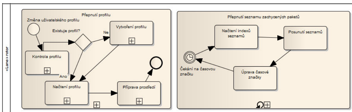
Obrázek 8 - Diagram činnosti vlákna "rotor"
