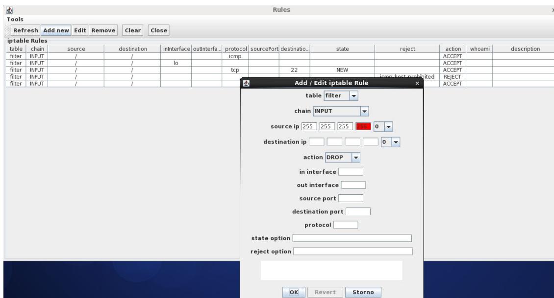
Obrázek 14 - Dialog pro přidání / úpravu pravidla pro firewall
