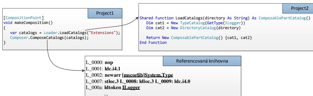
2-4 Z metody makeComposition je volána metoda LoadCatalogs v Project2 psaná ve Visual Basic a ComposeCatalogs ze zkompileované knihovny, dostupné pouze v MSIL instrukcích.
