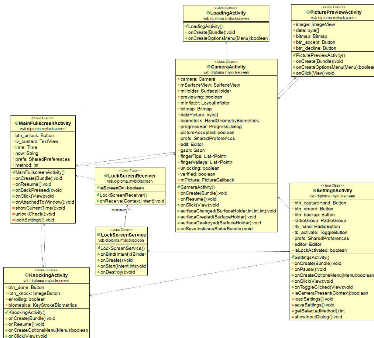
Obrázek 6-3: Třídní diagram aplikace
